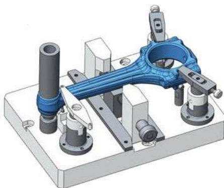
Készülék maráshoz
