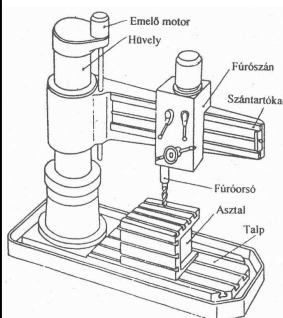
3.8. ábra Sugárfúrógép nézeti és kinematikai ábrája
