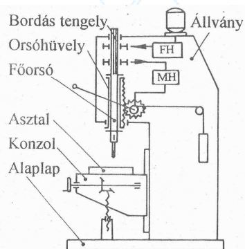
Oszlopos és állványos fúrógép felépítése
