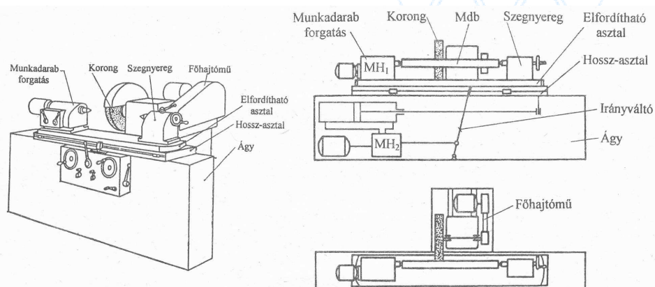
3.14. ábra Egyetemes palástköszörűgép nézeti és kinematikai ábrája
