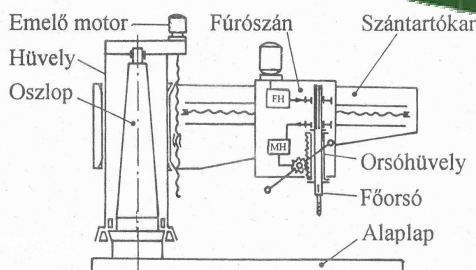
3.8. ábra Sugárfúrógép nézeti és kinematikai ábrája
