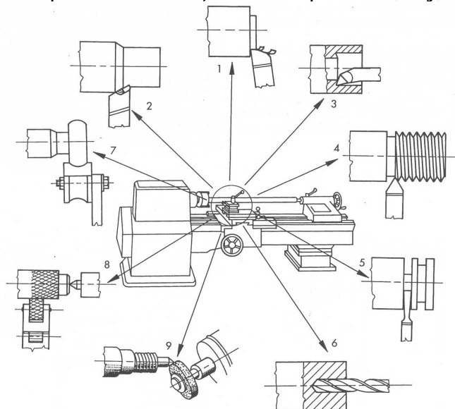
10.1. ábra. Jellegzetes esztergaműveletek
