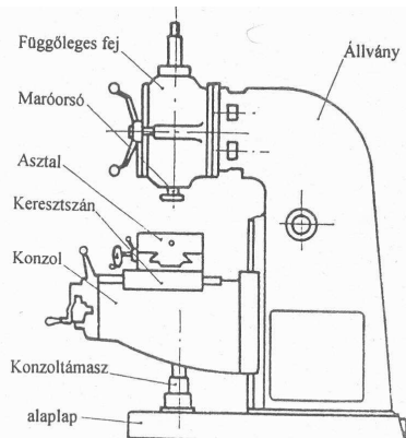
3.11. ábra Függőleges konzolos marógép
