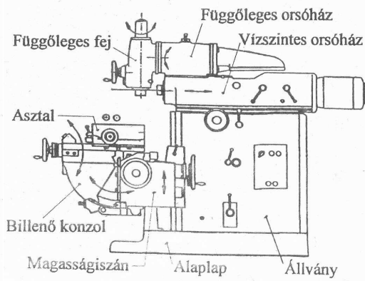
3.12. ábra Szerszámmarógép
