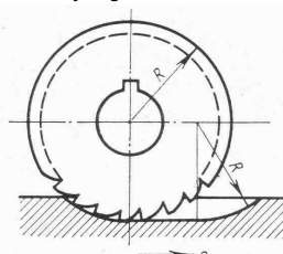
4-1. ábra. Ékhorony marása tárcsamaróval
