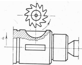
4-4. ábra. Íves reteszhorony marása tárcsamarával
