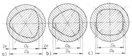
2.75. ábra. Poligon tengelykötésű profilok a) P3-profil b) P3C-profil; c) P4C-profil;
